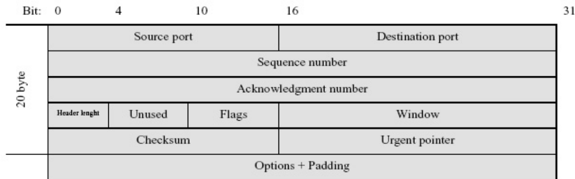
Slika 1.9. TCP header
